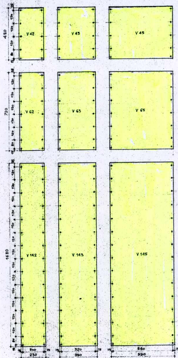
V-JOUES au FONDS VERTICAUX PERCEMENTS : TROUS \varnothing : 8 mm
