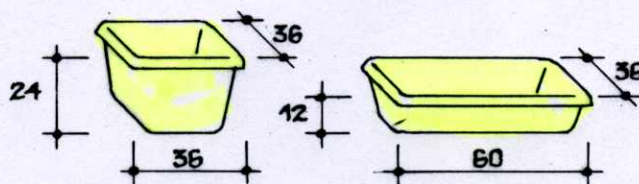
BACS/TIROIRS (POUR CASES 24/36/36 OU 12/60/36)
