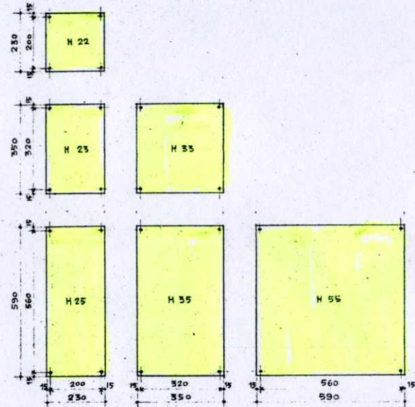
H-TABLETTES HORIZONTALES PERCEMENTS : TROUS \varnothing : 8 mm
