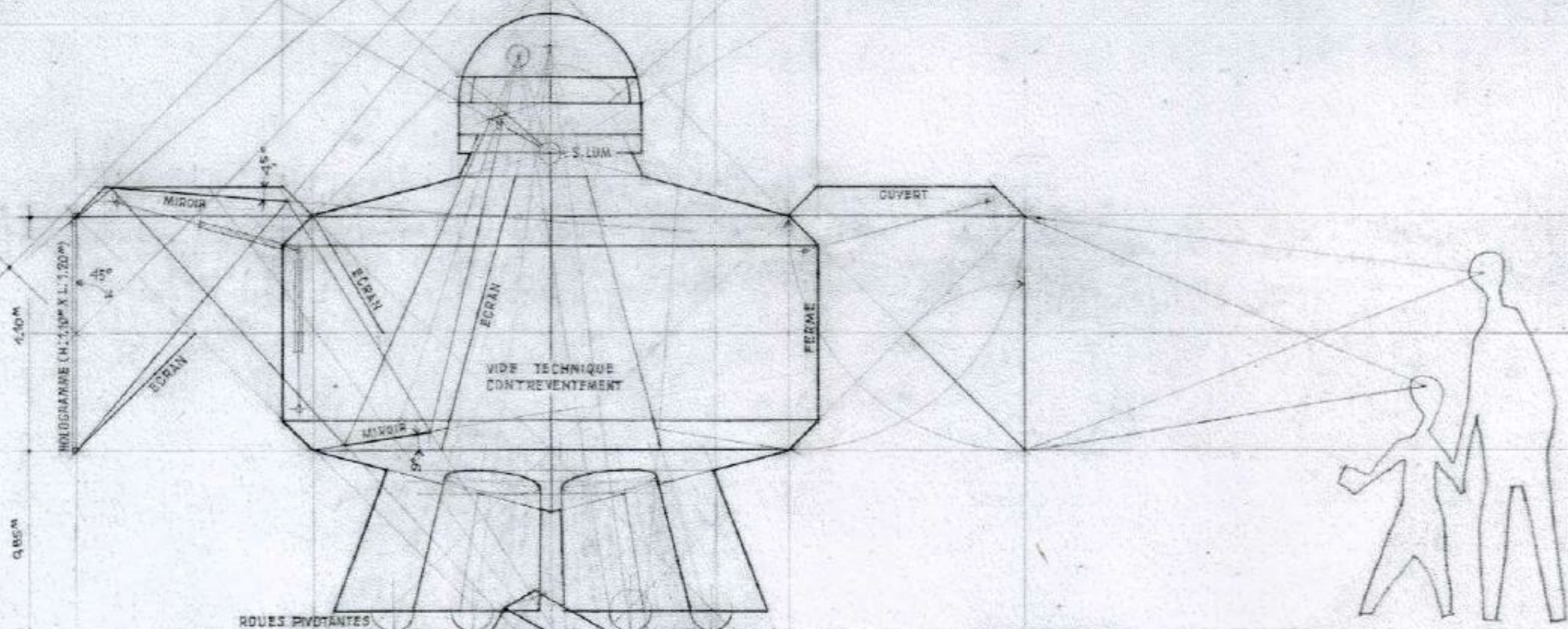
ELEVATION PROFIL
