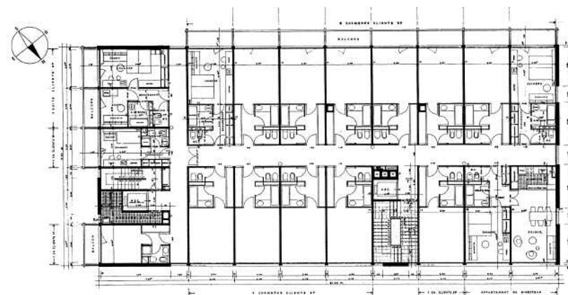
Niveau 1
