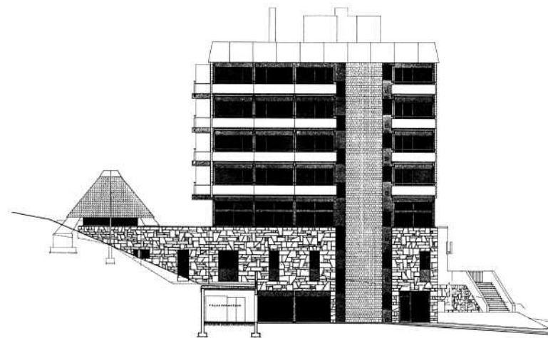
Façade est
