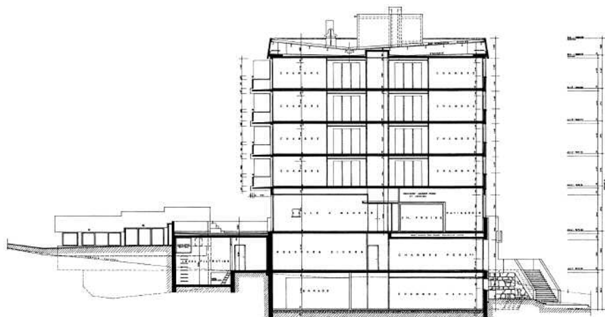
Coupe transversale AA
