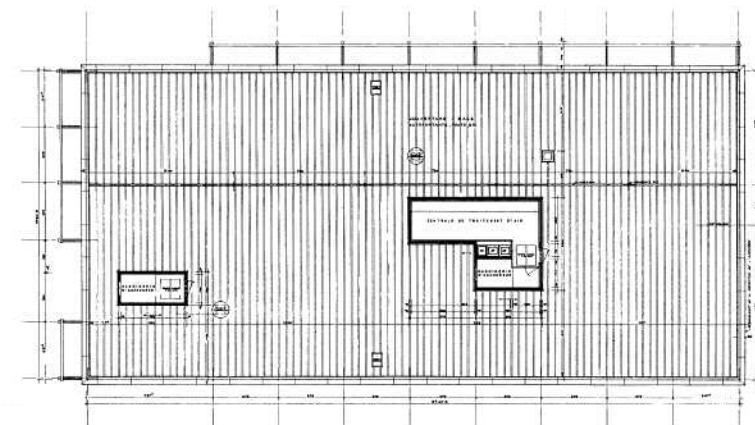
Toiture
