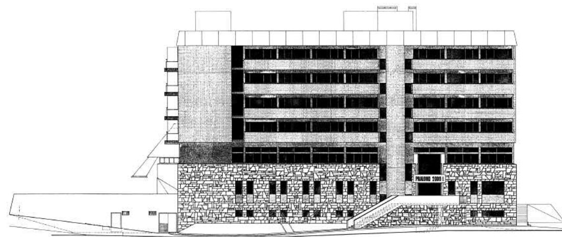
Façade Nord
