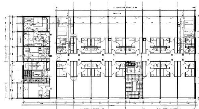
Niveaux 2, 3, 4
